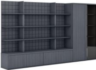
КОМПОНОВКА 10 Ш: 350 / Г: 48,5 / В: 200 СТЕНОВАЯ ПАНЕЛЬ ( АН501 ) - 2 ШТ. ТУМБА ( АН301 ) - 2 ШТ. ШКАФ С ПОЛКАМИ ( АН405 ) - 1 ШТ. ШКАФ - ГАРДЕРОБ ( АН402 ) - 1 ШТ.
