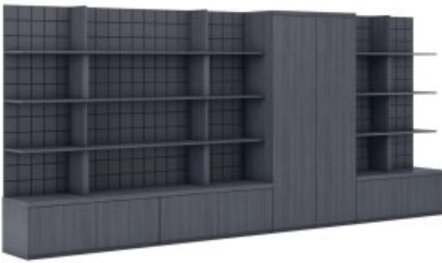
КОМПОНОВКА 11 Ш: 470 / Г: 48,5 / В: 200 СТЕНОВАЯ ПАНЕЛЬ ( АН501 ) - 3 ШТ. ТУМБА ( АН301 ) - 3 ШТ. ШКАФ С ПОЛКАМИ ( АН401 ) - 1 ШТ. ШКАФ - ГАРДЕРОБ ( АН402 ) - 1 ШТ.
